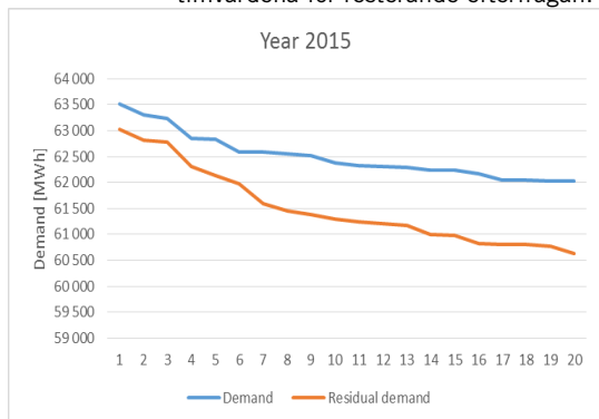
Figur 5.2 Varaktighetskurvor för året 2015
