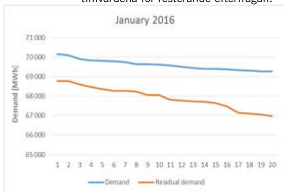
Figur 5.1 Varaktighetskurvor för januari 2016
